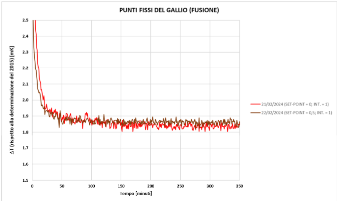
Figura 18: Plateau eseguiti senza effettuare misurazioni sulla termocoppia differenziale
