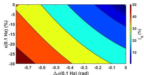
Fig.2: \xi_g vs errore di rapporto e fase del TV in presenza di f_{sub-h} a 6 Hz e f_{sub-h,out} a 4.9 Hz
