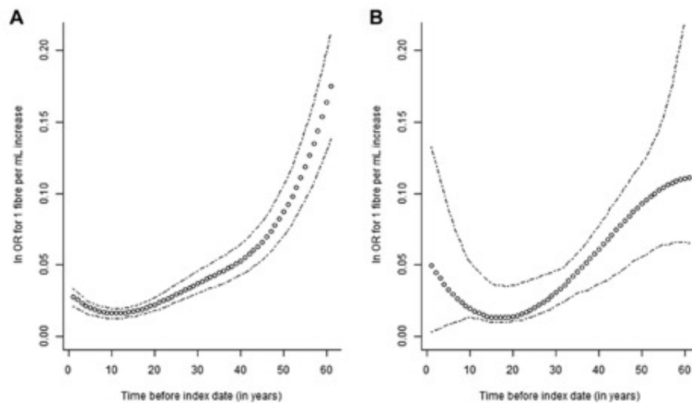
Figura 2. Stima log OR del mesotelioma pleurico associata a un incremento di una fibra per millilitro nella dose quotidiana di esposizione all'amianto mediata annualmente per t anni prima della diagnosi/intervista aggiustata per l'intensità ricevuta in altri anni, anno di nascita ed età alla diagnosi/intervista. (A) Risultati ottenuti con i dati del caso-controllo francese raccolti in Lacourt et al. (B) Risultati ottenuti usando i dati dello studio caso-controllo francese 1998-2005 41 [trad. dell'autore].
